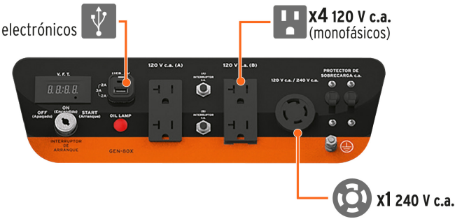
Páneles de control GEN-80X
