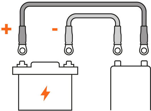
Conexión de batería a inversor
